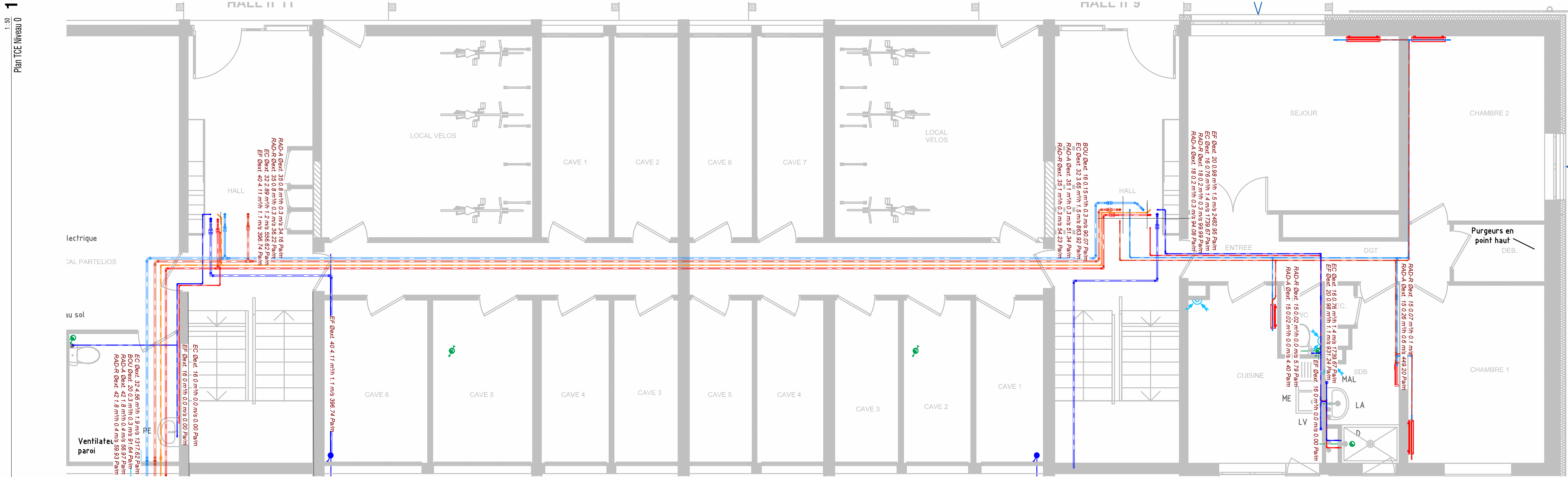
1 Plan TCE Niveau 0 1:30
