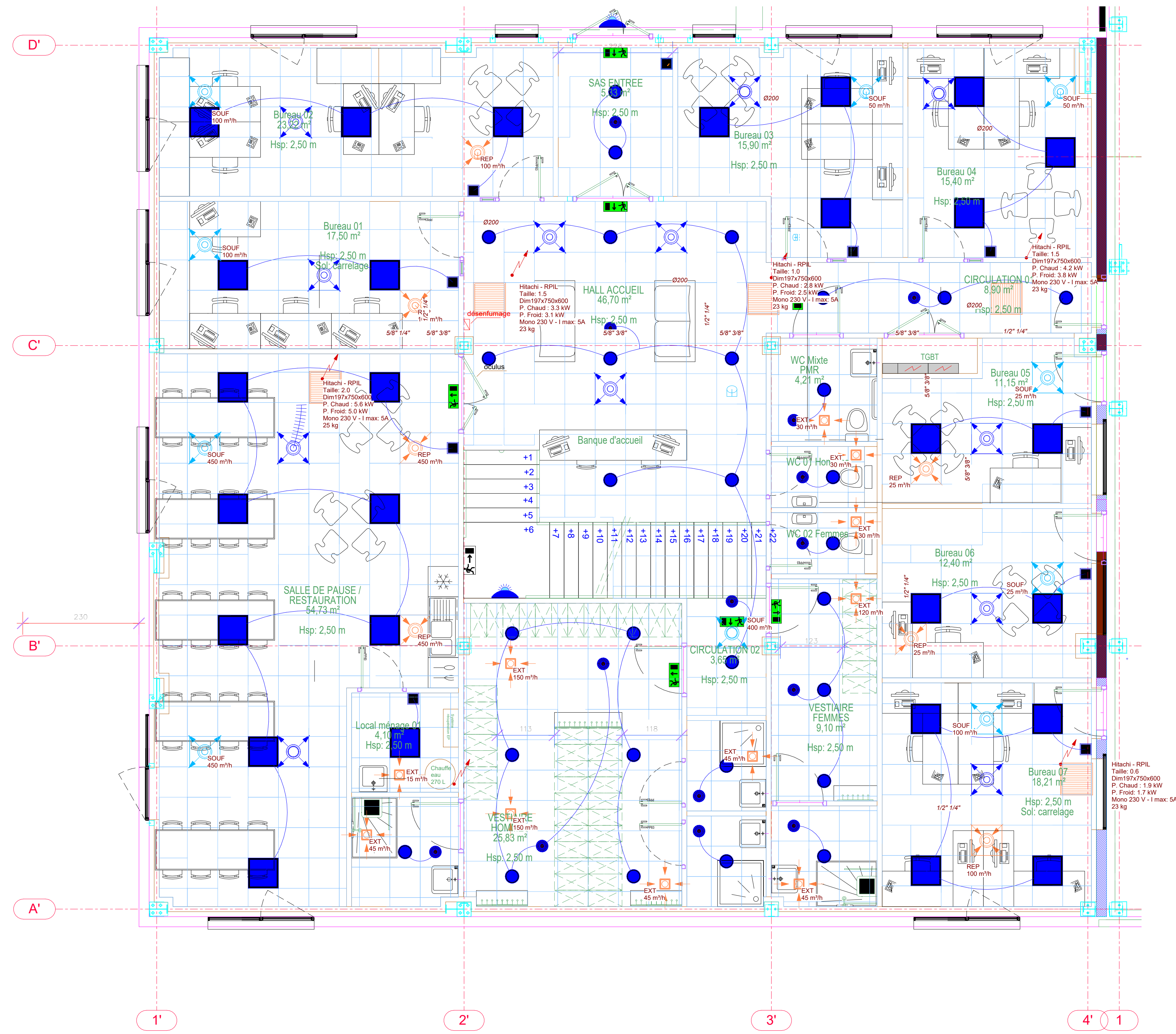
4 Plan CVC Niveau 0 1:30
