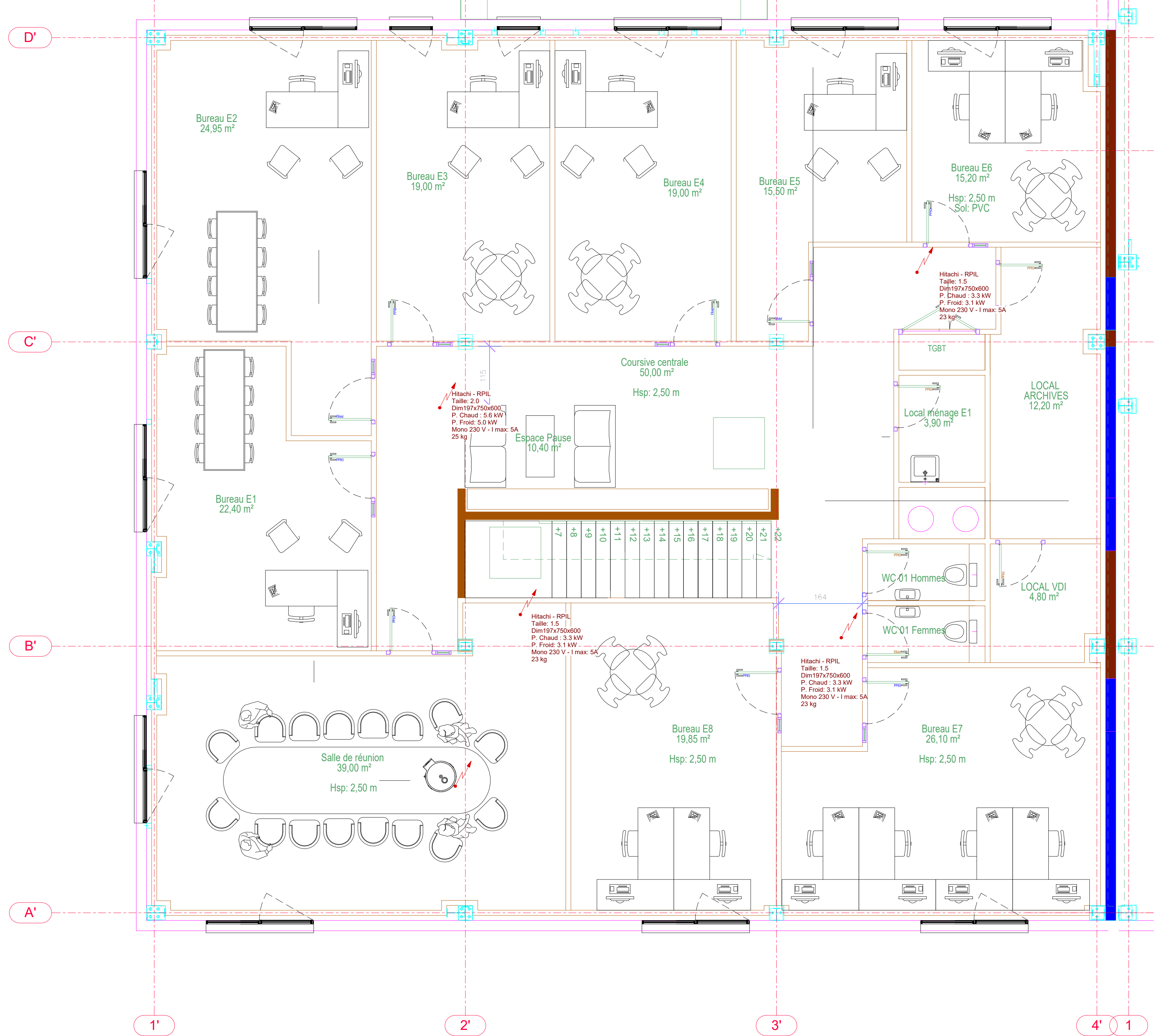
2 Plan ELEC Niveau 1 1:30
