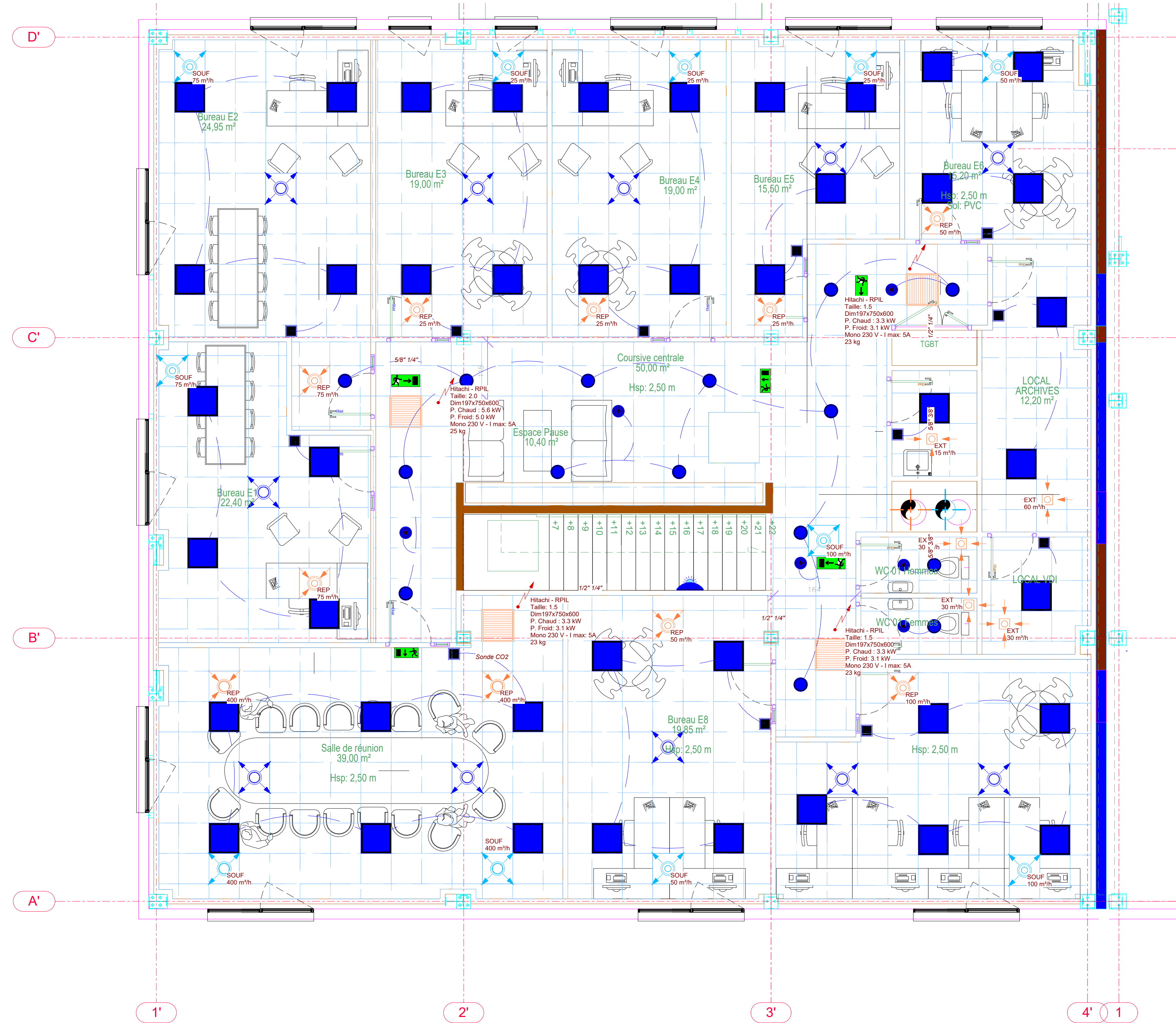
3 Plan CVC Niveau 1 1:30
