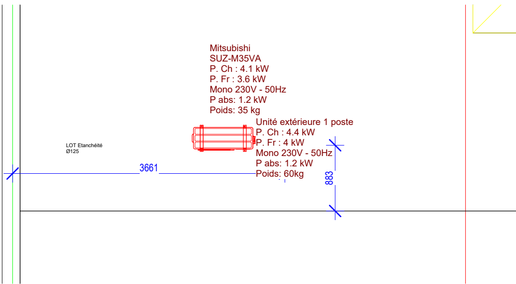
2 Plan Niveau 2-CVC - Bureau de quai 01 1:50
