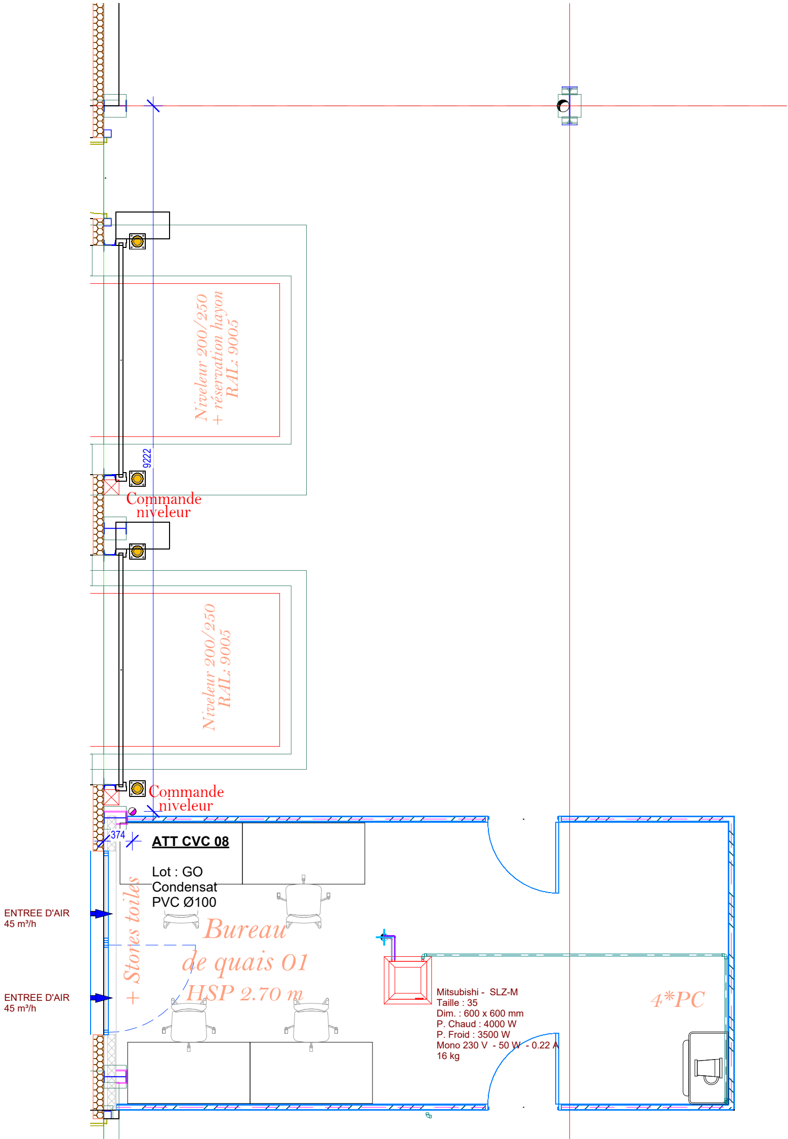
1 Plan CVC Niveau 0 1:50
