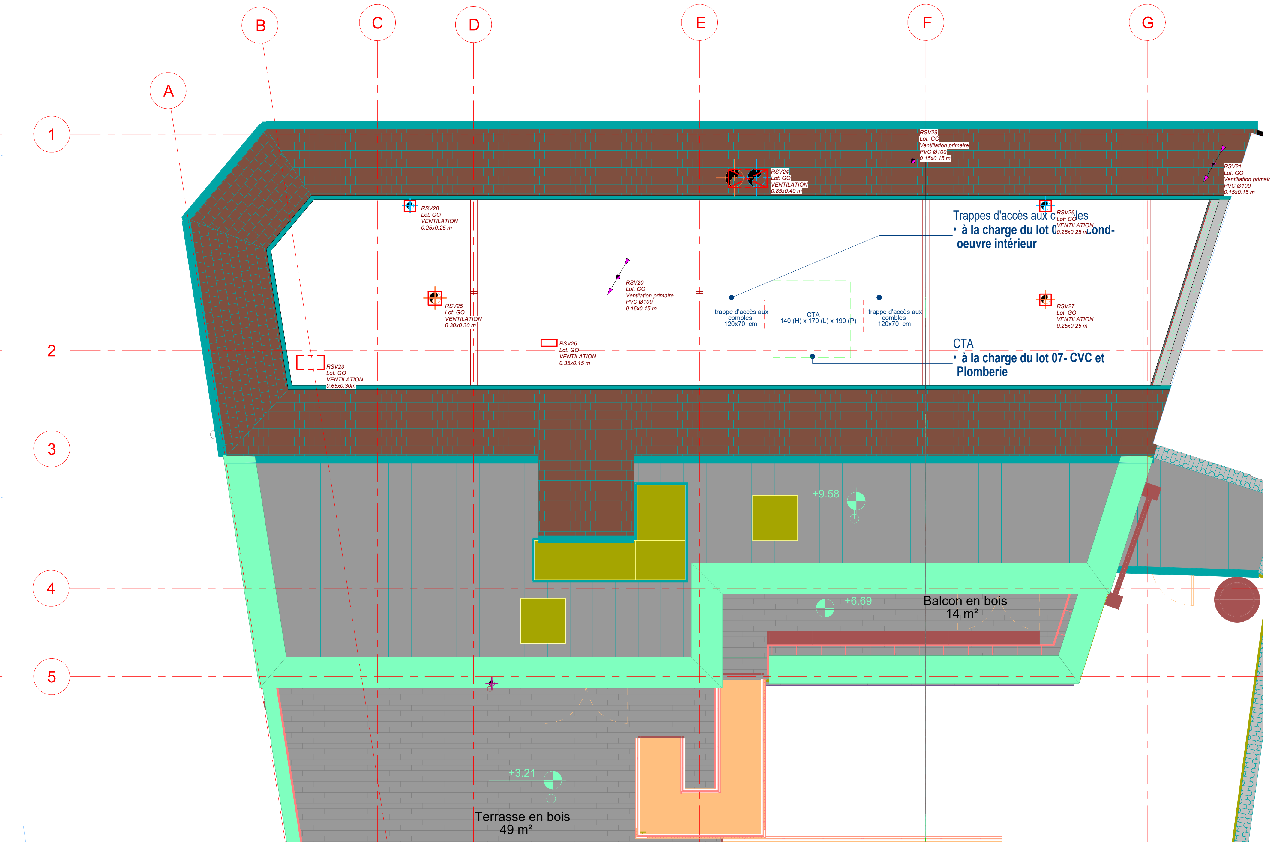
4 Plan Niveau 3:TOC Copie 1 1:50
