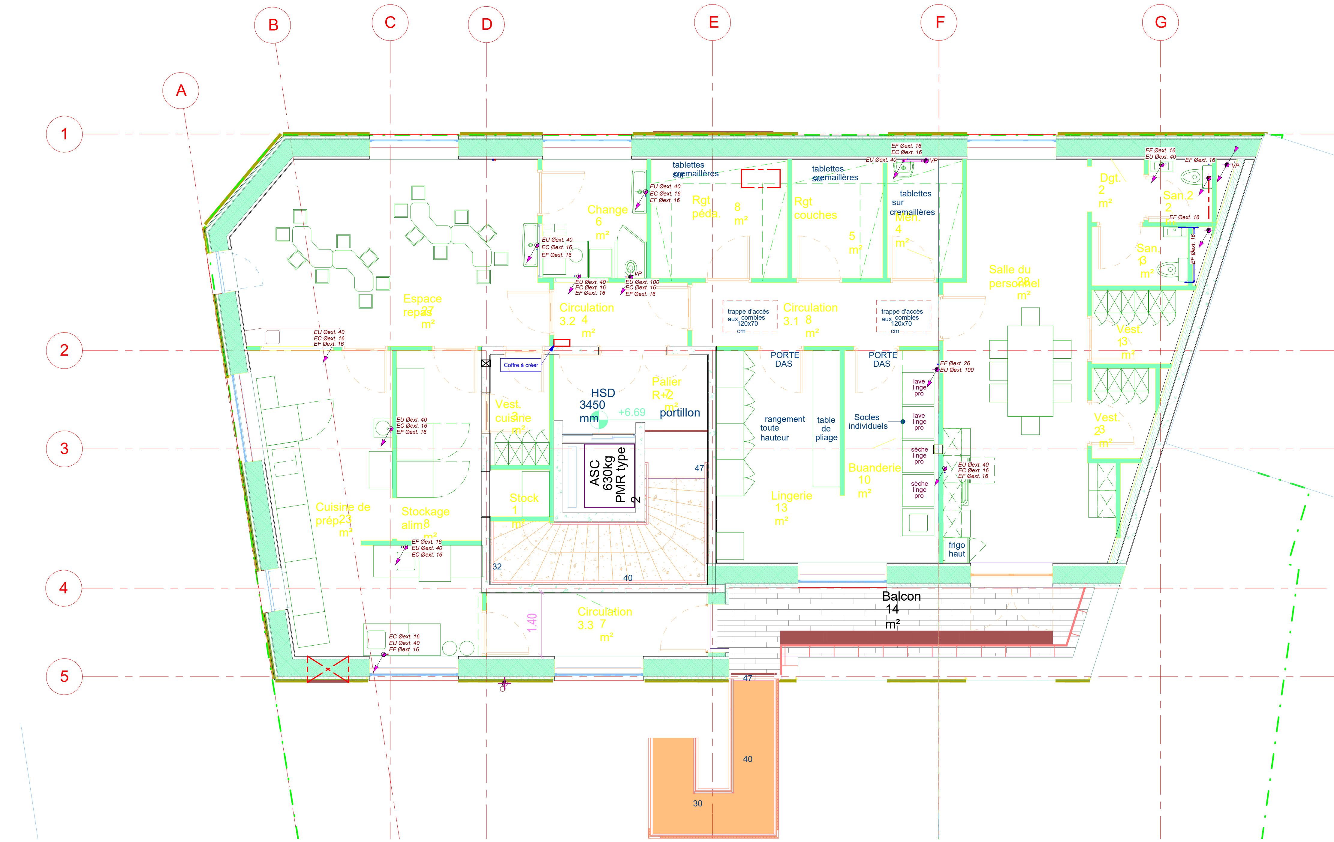
3 Plan Niveau 2:TOC 1:50
