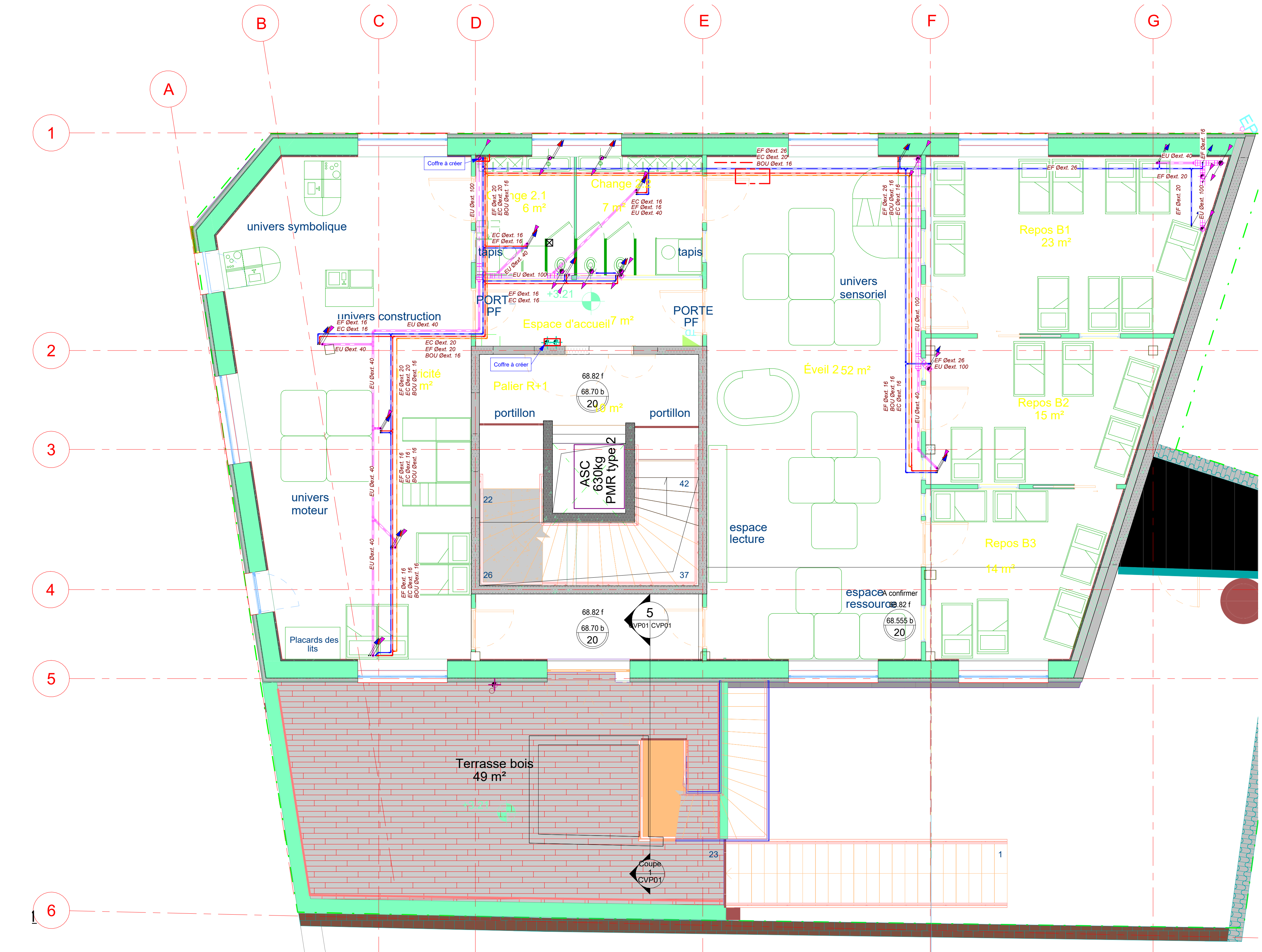
2 Plan TOC Niveau 1 1:50
