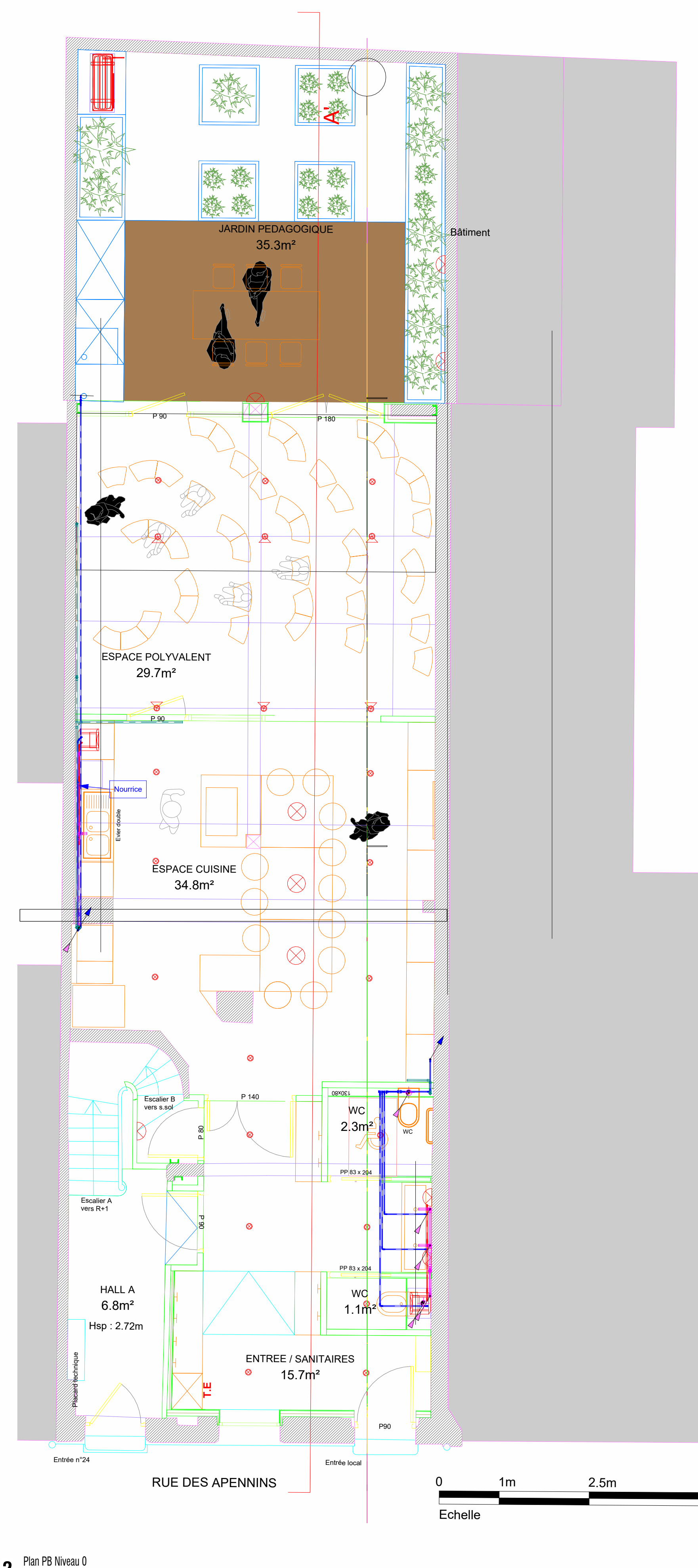
2 Plan PB Niveau 0 1:50
