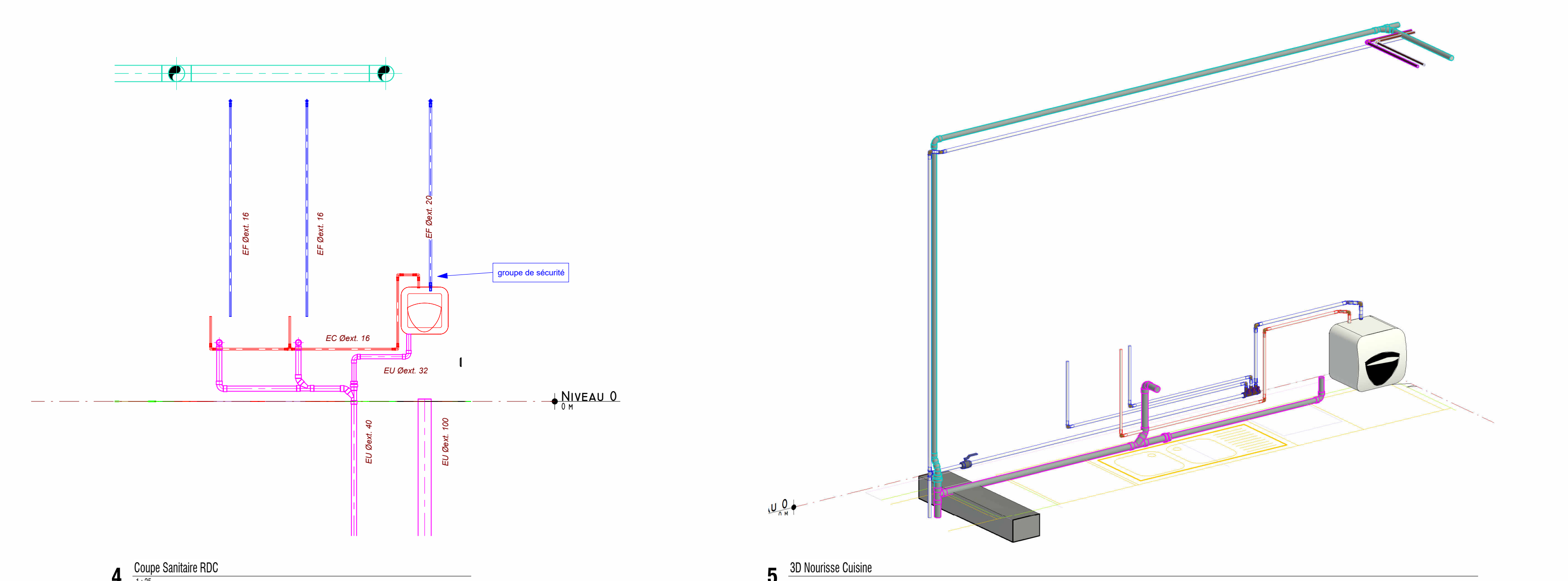
4 Coupe Sanitaire RDC 1:20
